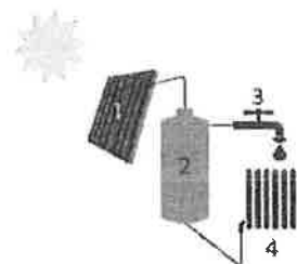
1. Zonnecollector | 2. Opslagvat zonneboiler | 3. Sanitair warm water | 4. Afgegeven element voor ruimteverwarming (optioneel)
